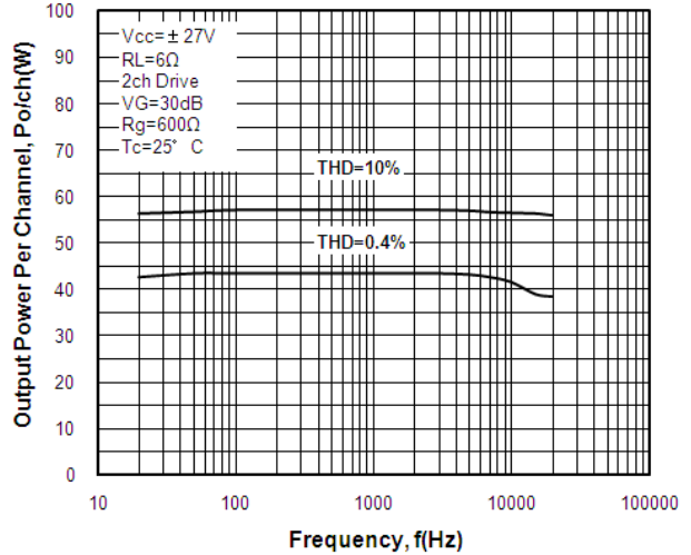
Po-f
