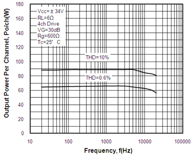
Po-f STK433-890N-E
