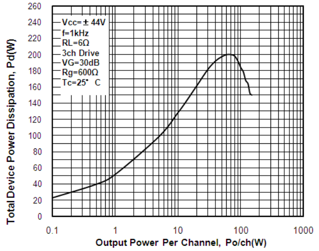
Pd-Po STK433-330N-E
