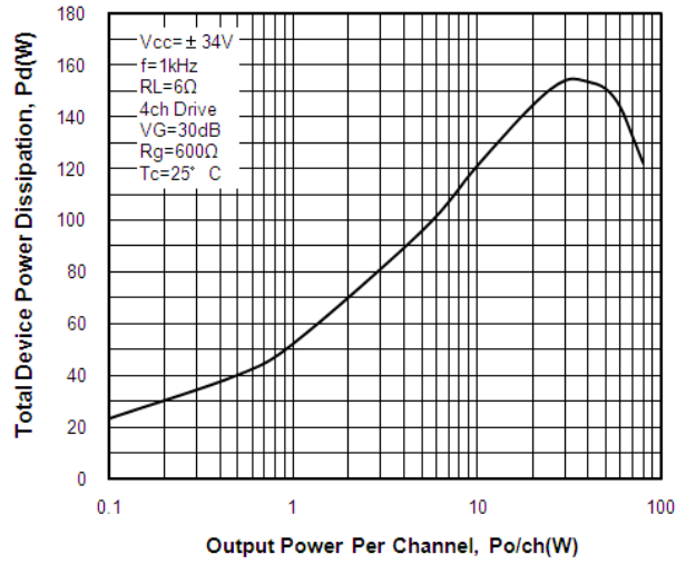
Pd-Po STK433-890N-E
