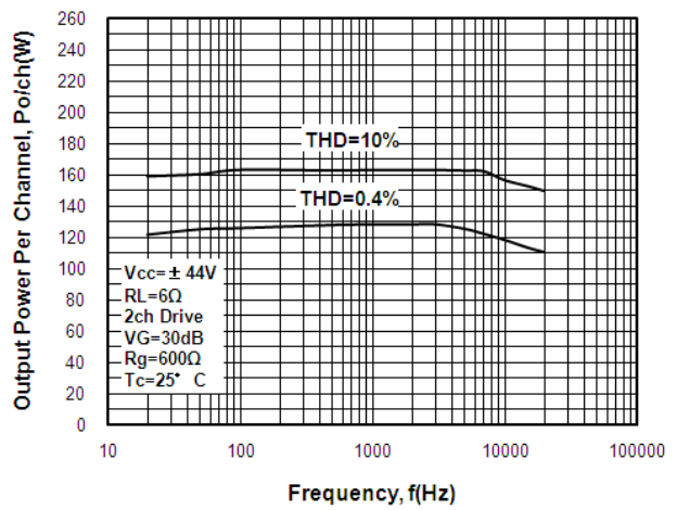
Po-f
