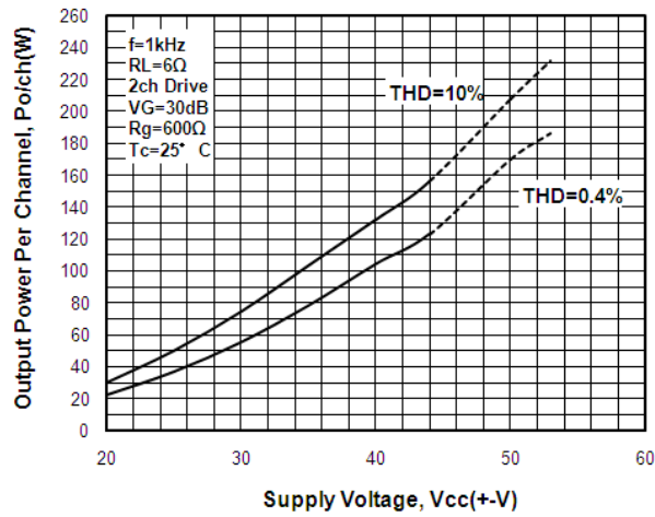
Po-Vcc
