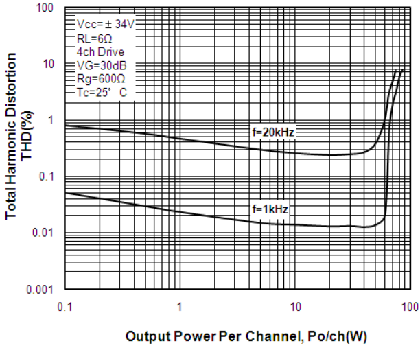
THD-Po STK433-890N-E
