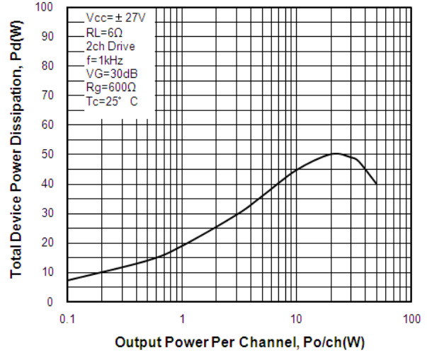
Pd-Po
