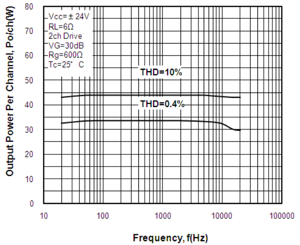
Po-f STK433-040N-E
