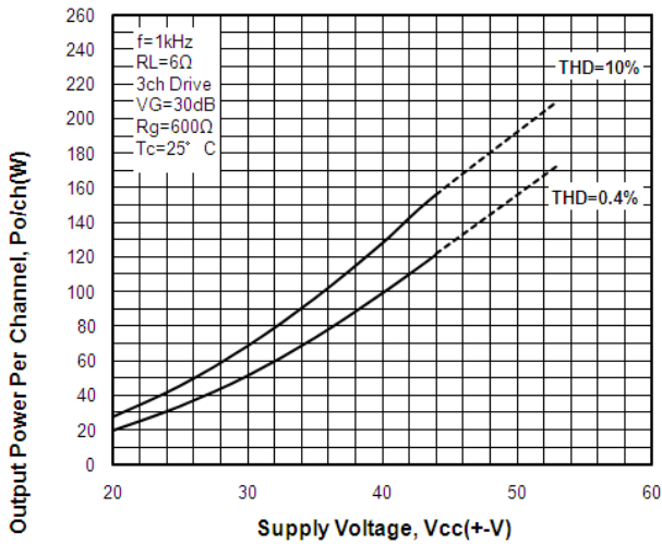
Po-Vcc STK433-330N-E
