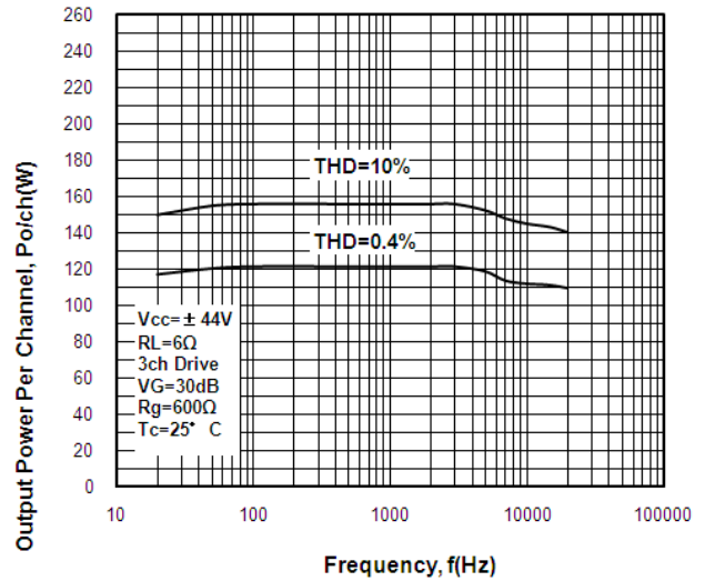
Po-f STK433-330N-E
