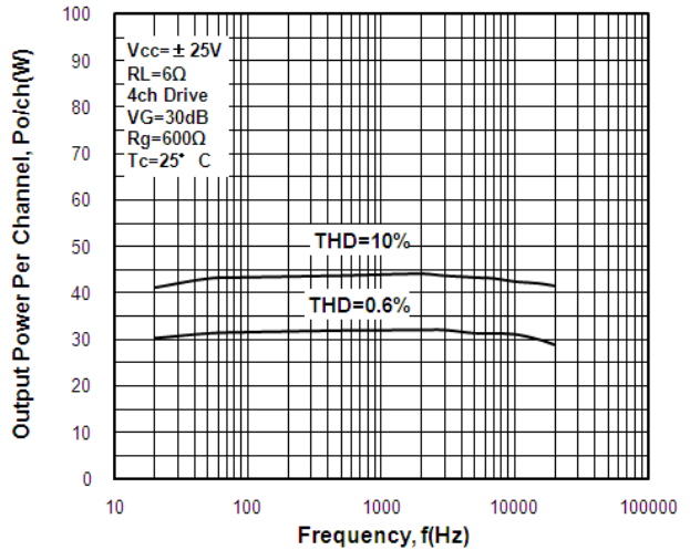
Po-f STK433-840N-E
