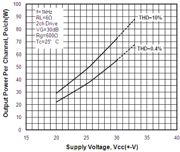
Po-Vcc
