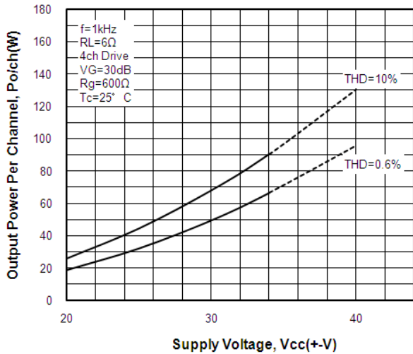
Po-Vcc STK433-890N-E
