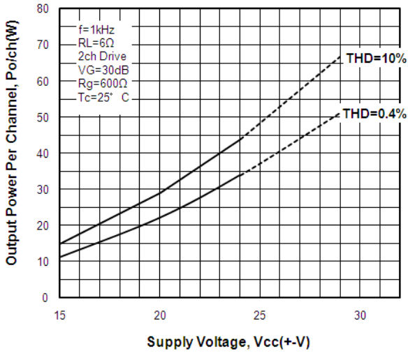
Po-Vcc STK433-040N-E
