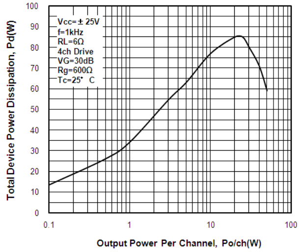
Pd-Po STK433-840N-E
